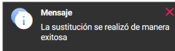
Figura 3.7 Mensaje
